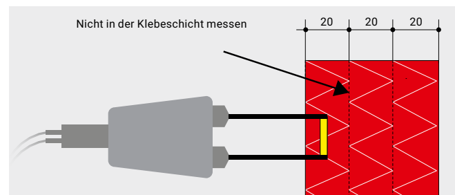
Richtige Messergebnisse mit isolierten Elektroden in der Holzfaser-Dämmplatte (bei Nassplatten)
