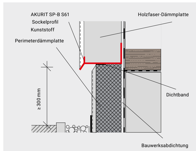
Sockeldetail mit AKURIT SP-B S61 Sockelprofil Kunststoff
