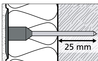
Die „Verankerungslänge“ muss 25 mm betragen
