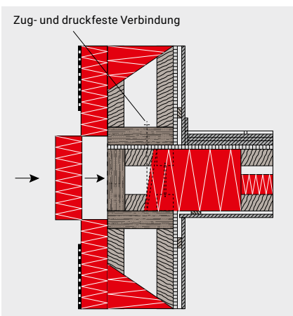
Setzungssicherer Geschossstoß
