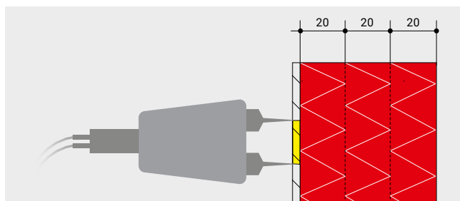
Falsche Messergebnisse bei Oberflächenfeuchte (Regen, Tau)
