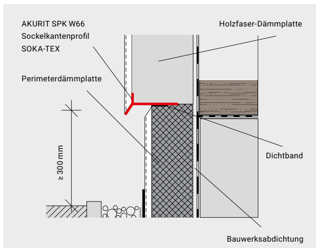
Sockeldetail mit AKURIT SPK W66 Sockelkantenprofil SOKA-TEX
